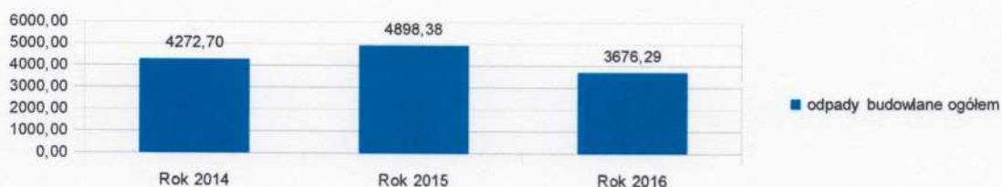
Wykres 10. Zestawienie ilości odebranych odpadów budowlanych i rozbiórkowych stanowiących odpady komunalne łącznie na przestrzeni lat 2014-2016 r. [Mg].
