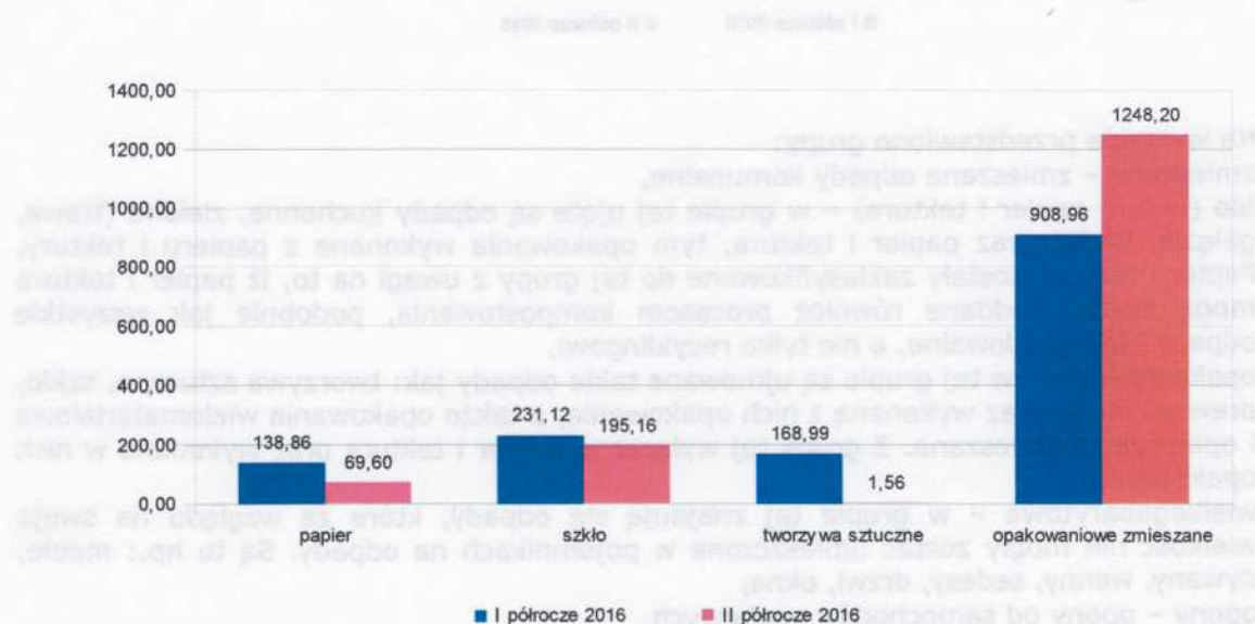
Wykres nr 2. Zestawienie ilości odebranych odpadów selektywnie zebranych – surowcowych w 2016 r. [Mg].
