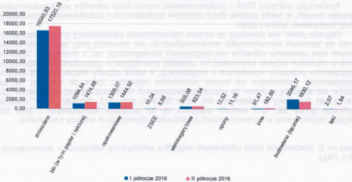
Wykres nr 1. Zestawienie ilości odpadów komunalnych odebranych z nieruchomości w podziale na grupy w roku 2016 [Mg].
